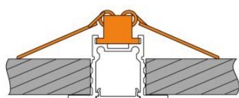
Profileinbaufeder Deckenausschnitt 26mm Einbautiefe 35/70mm
