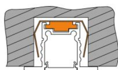
Profilbefestigungsklammer Deckenausschnitt 26mm Einbautiefe 30mm
